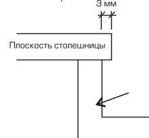
Рис.1 Приклейка мойки под столешницу с полировкой выреза
